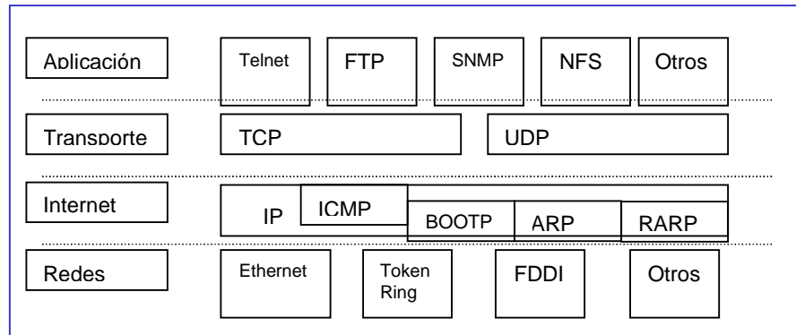
Figura no. 1. Descripción del modelo DOD y su referencia con TCP/IP
