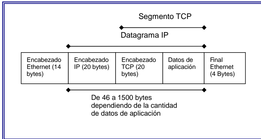
Figura no. 3. Un frame Ethernet con los encabezados de todos los componentes de un paquete TCP
