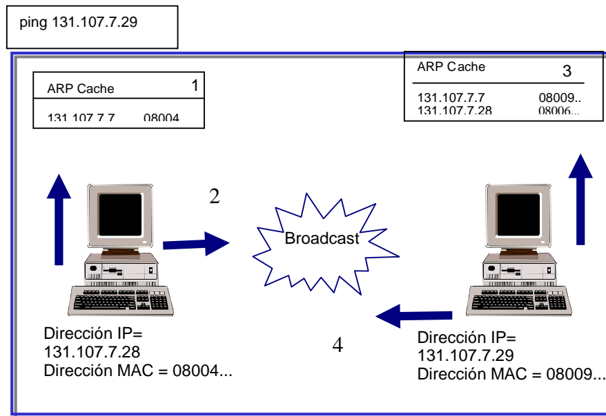
Figura no. 5. Proceso de resolución de direcciones en una red remota
