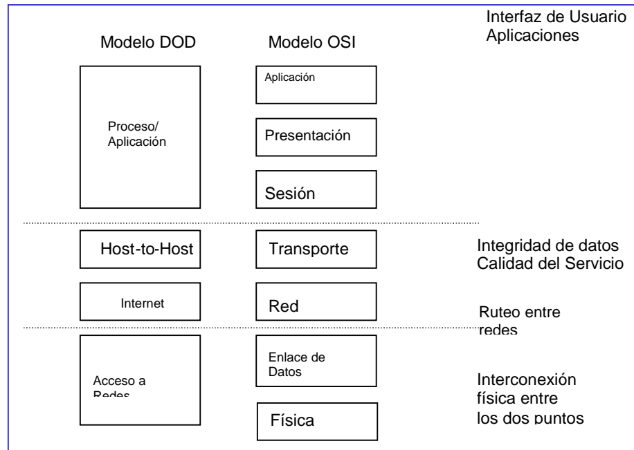
Figura no. 2. Cuadro comparativo entre el Modelo DOD y el Modelo OSI
